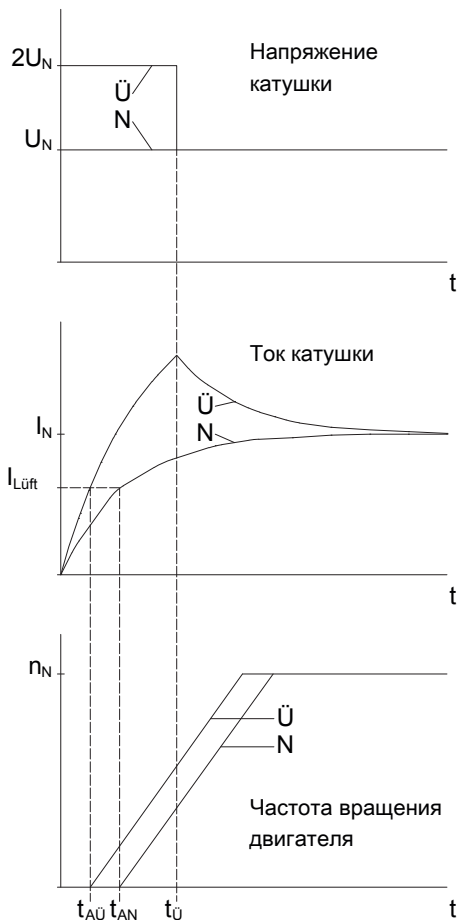
Рис. 2. Принципиальные кривые напряжения катушки, тока катушки и частоты вращения двигателя при нормальном возбуждении (N) и форсированном возбуждении ( \ddot{U} )
