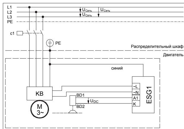
Рис. 8. Питание выпрямителя от клеммника электродвигателя или клеммного блока КВ (см. раздел «Подключение выпрямителя к клеммнику двигателя или клеммному блоку КВ»).
