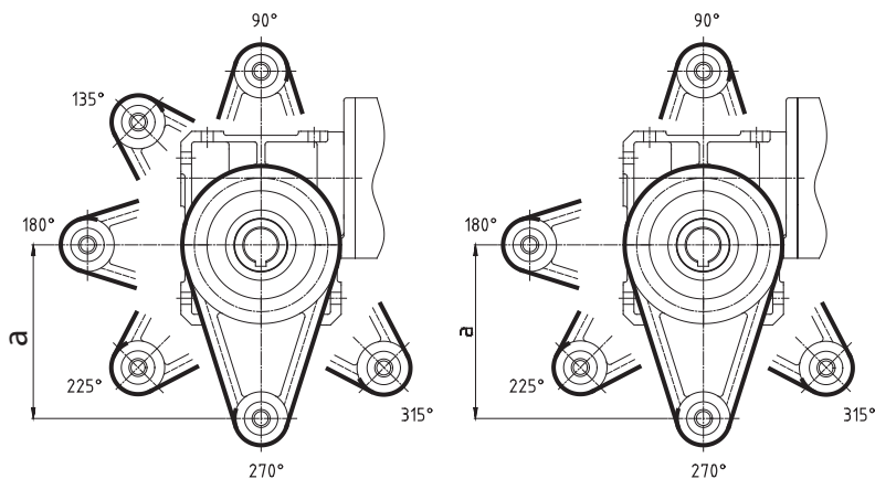
DA/I 90 .. DA/I 315
