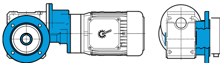
SK 1SI 63/H10 FA/I IEC71 - 71 L/4 Полый вал, Фланец, сторона А, червячный мотор-редуктор с цилиндрической предступенью Т1
