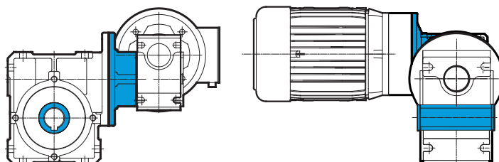
SK 1SI 75/40 IEC80 - 80 SH/4 Полый вал, Сдвоенный червячный мотор-редуктор U1, Положение клеммной коробки КК1
