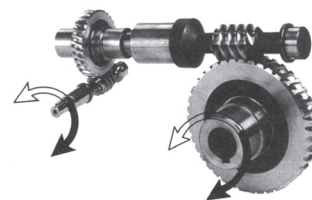
NMRV+NMRV - NRV+NMRV
